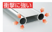
脚部断面図
