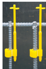
LP-1013 径10・13mm兼用
