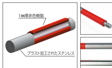
強固な ジョイント部
