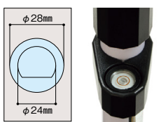
水準器(本体一体) 40'/2mm (PP-200EVのみ)
