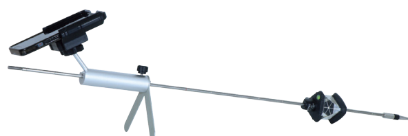
プレート型二脚がスマートフォンとプリズムを保護
