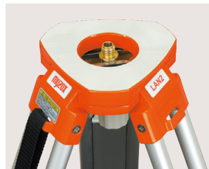
LAN2-OL 平面脚頭定芯棒 5/8インチ
